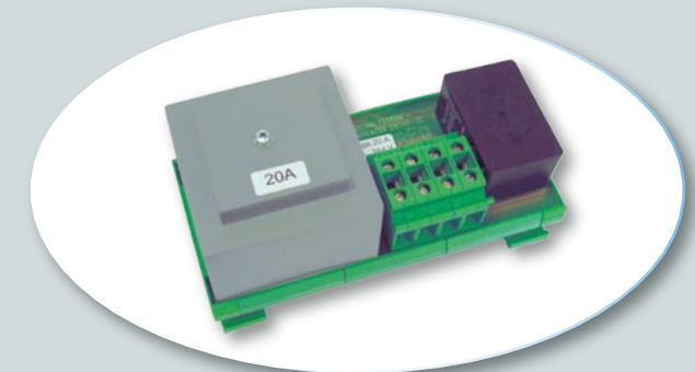
Reihe ED 746 Einschalt - Strombegrenzer Kompakte Bauform. Max. 32 A.
